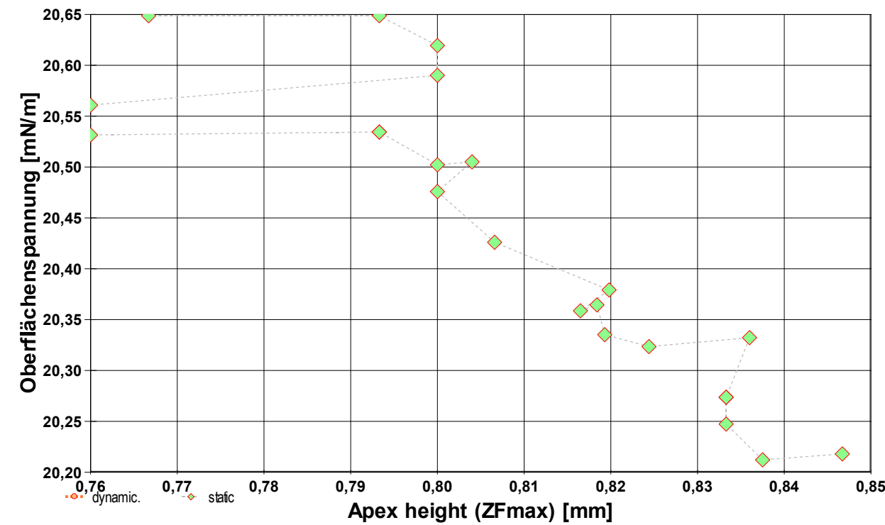
- Diagramm 2. Lamellenhöhe in Abhängigkeit von der Oberflächenspannung - 'Lamellenhöhen' 21
